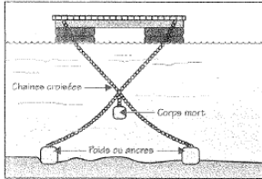
Figure 18 : Ancrage d'un quai
